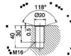
PRZEKRÓJ MOCOWANIA NA GWINT
