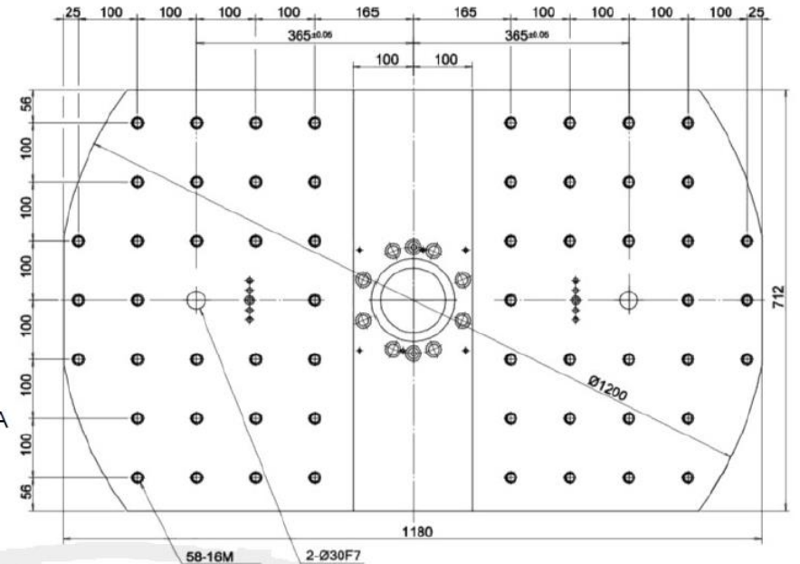
PRZEKRÓJ MOCOWANIA NA GWINT
